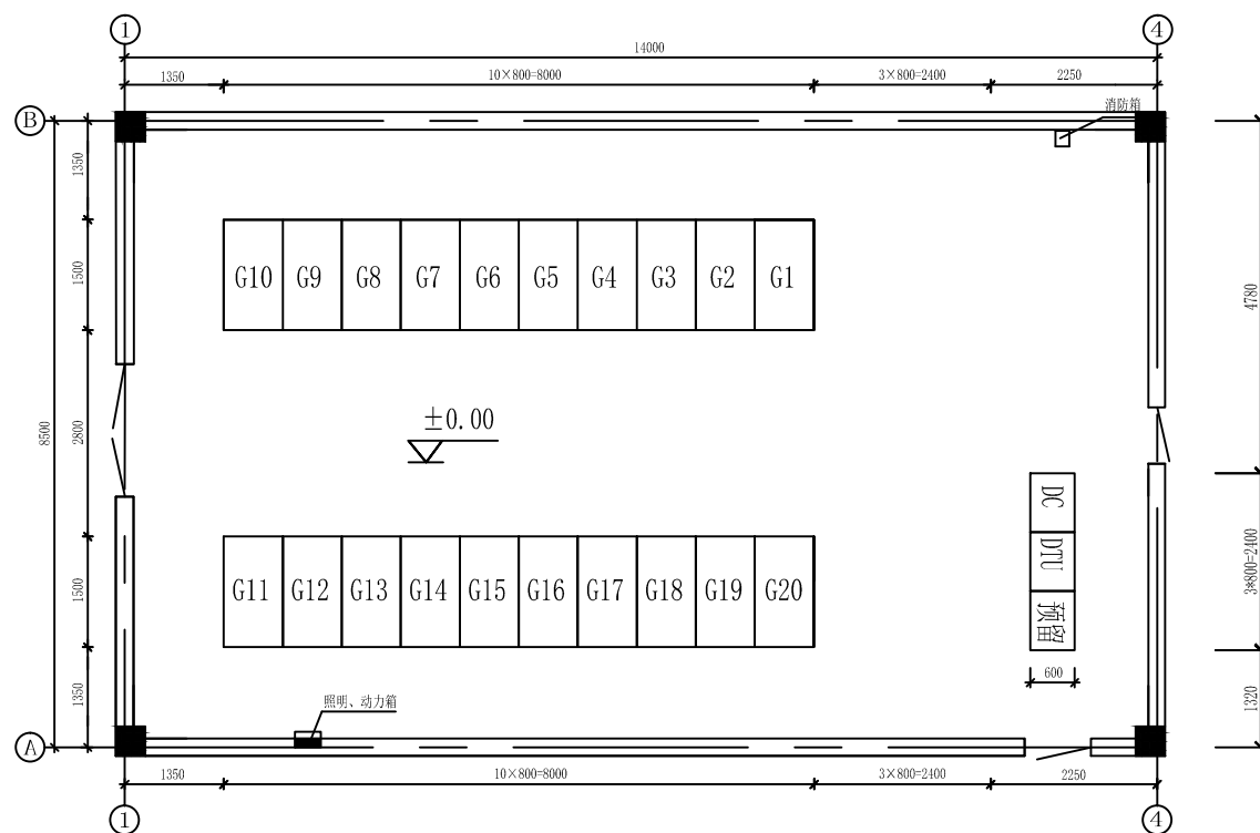
开闭所平面布置图
