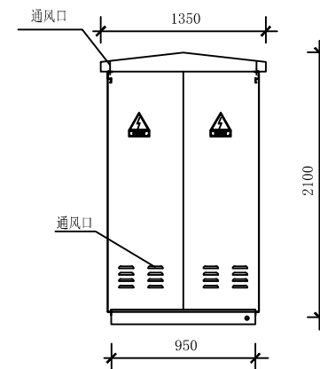
侧视图
