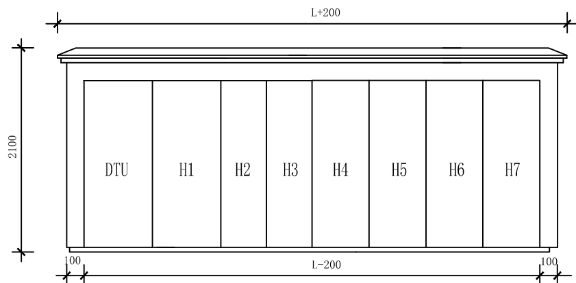
正视图
