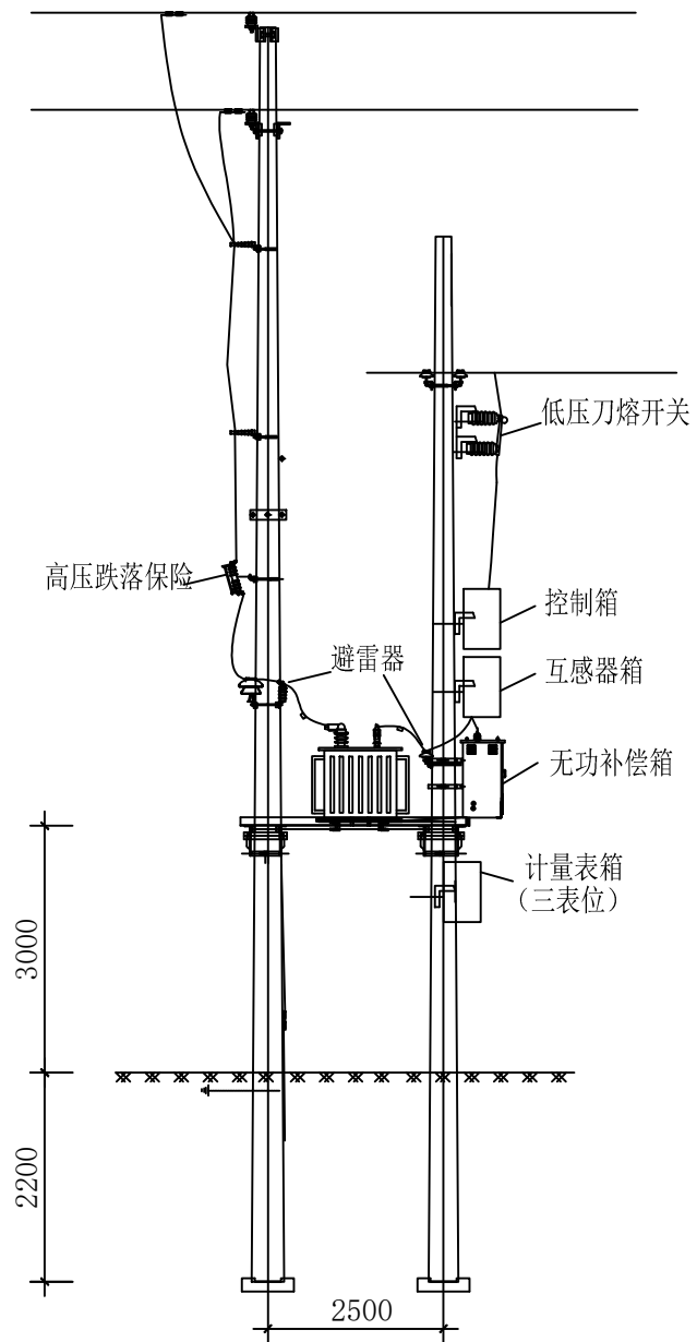
图2-2 200~250kVA柱上变压器安装示意图（低压计量）
