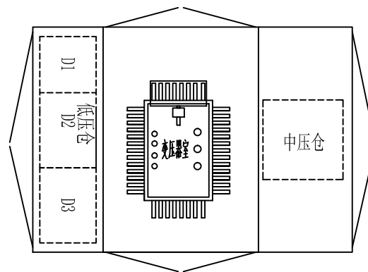
平面俯视图(油式)
