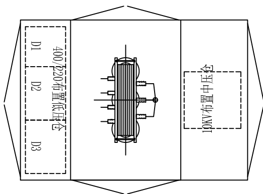
平面俯视图(干式)
